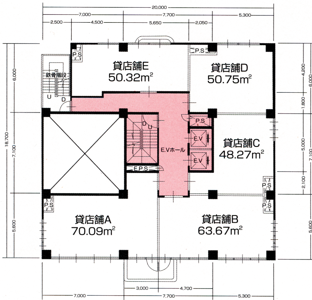
2階平面図
