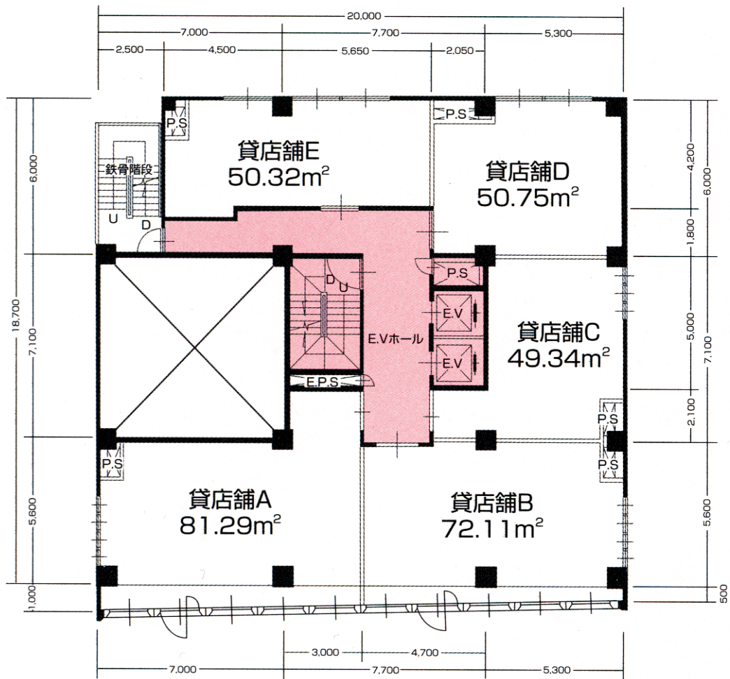
3～6階平面図
